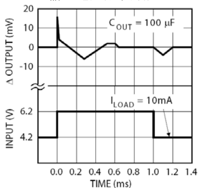
输入电压触发响应
