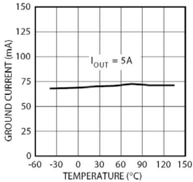
对地电流 VS 温度
