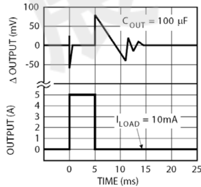
负载响应
