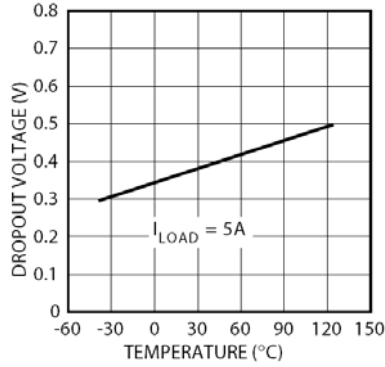
压差 VS 温度
