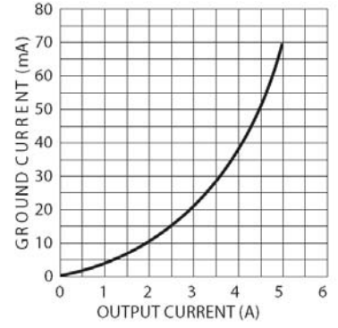
对地电流 VS 输出电流
