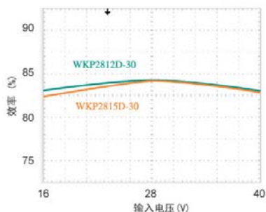
4: 输入电压-效率
